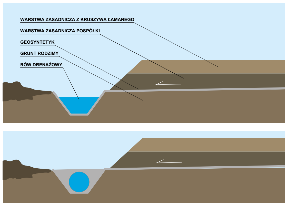
Rysunek 3. Przykładowy układ warstw platformy roboczej
