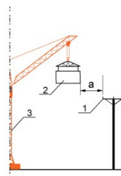
a - odległość pozioma między skrajnym przewodem linii a najbliższym elementem maszyny lub podnoszonego elementu budowlanego 1 - skrajny przewód linii elektroenergetycznej 2 - podnoszony element budowlany 3 - żuraw
